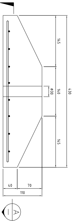
MUERTO TIPO IV ESC. 1:40
